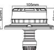
WL401PRO-LP
